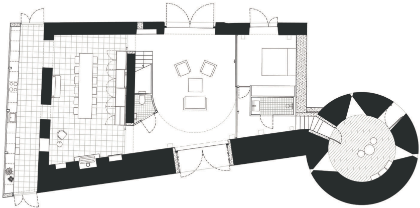
Réhabilitation d’une grange et d’anciens vestiges de château en habitation, à Montaut (47) — Plan RDC, 2021. © Seconde ligne
